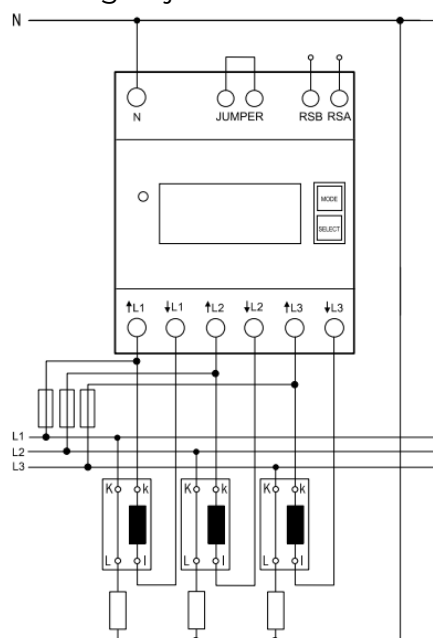
Koblingsskjema TN
