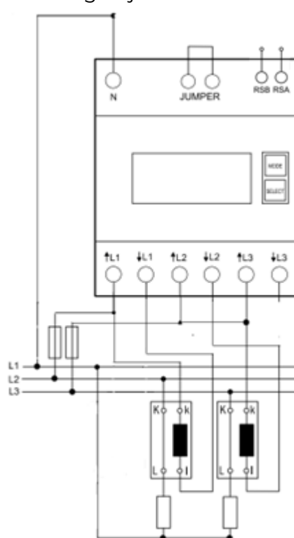
Koblingsskjema IT
