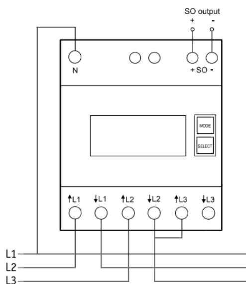
Koblingsskjema IT
