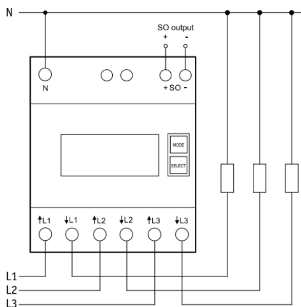
Koblingsskjema TN
