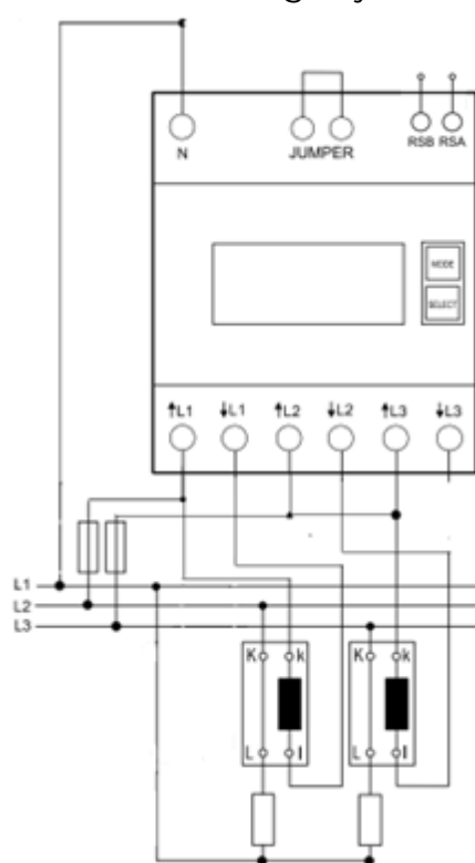
Koblingsskjema IT
