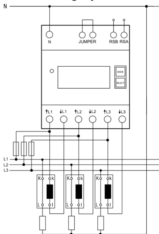
Koblingsskjema TN
