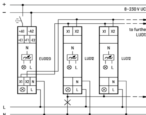
Koblingsskjema for 1 sone forkant dimming
