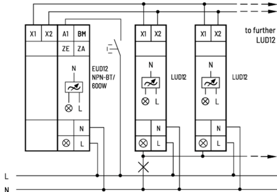
Koblingsskjema for flere sone forkant dimming
