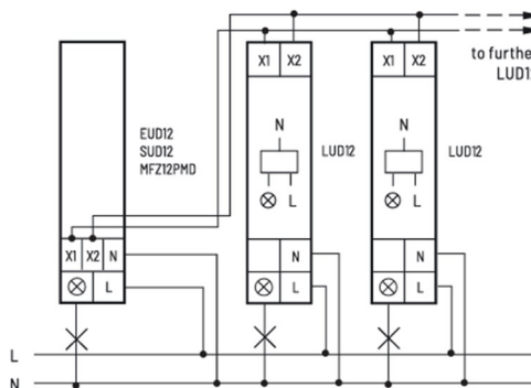
Koblingsskjema for flere soner. Bakkant dimming.
