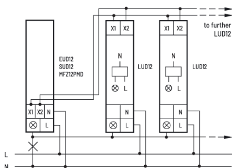
Koblingsskjema for 1 sone. Bakkant dimming
